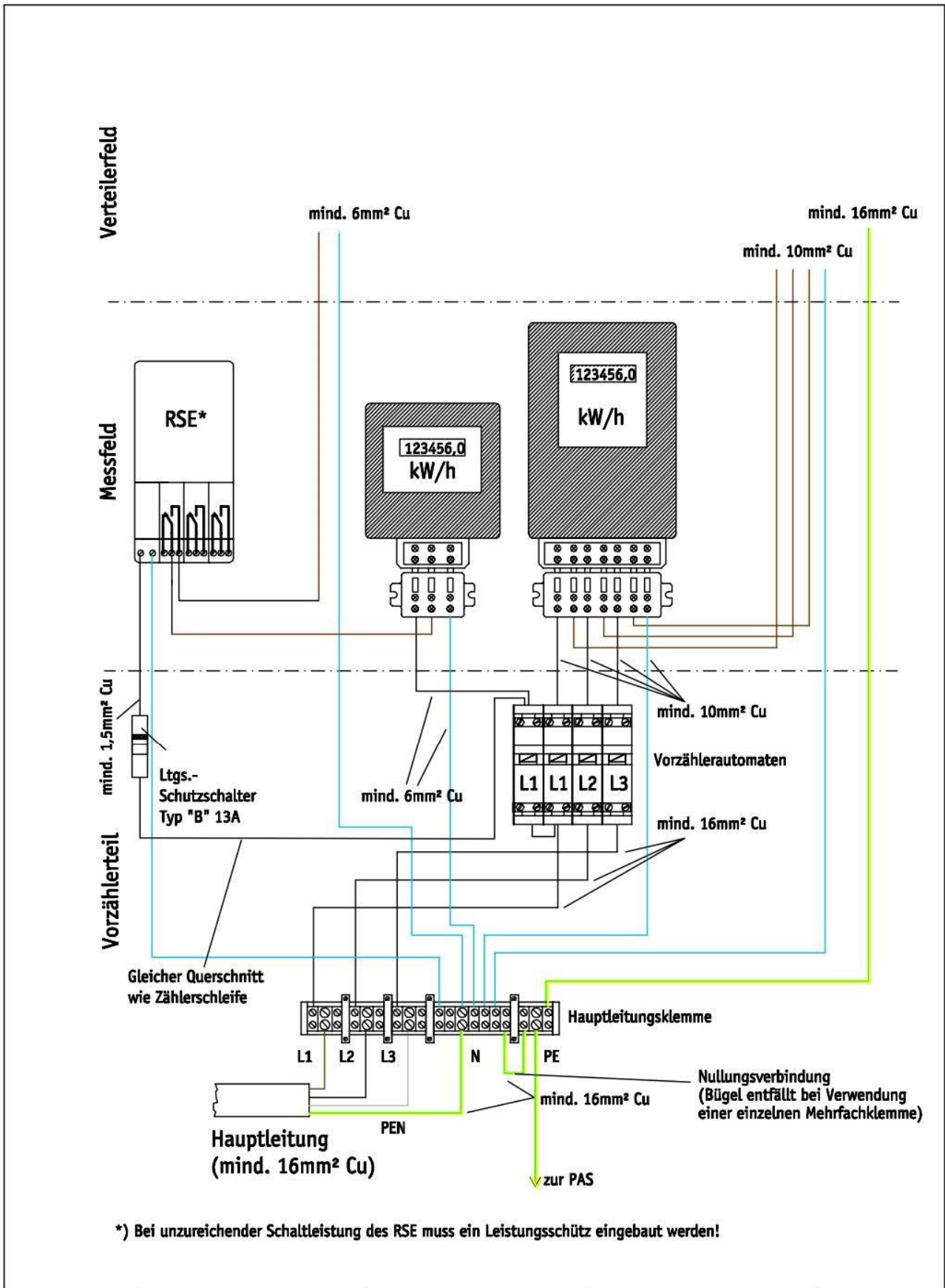
Verdrahtung Messeinrichtung
