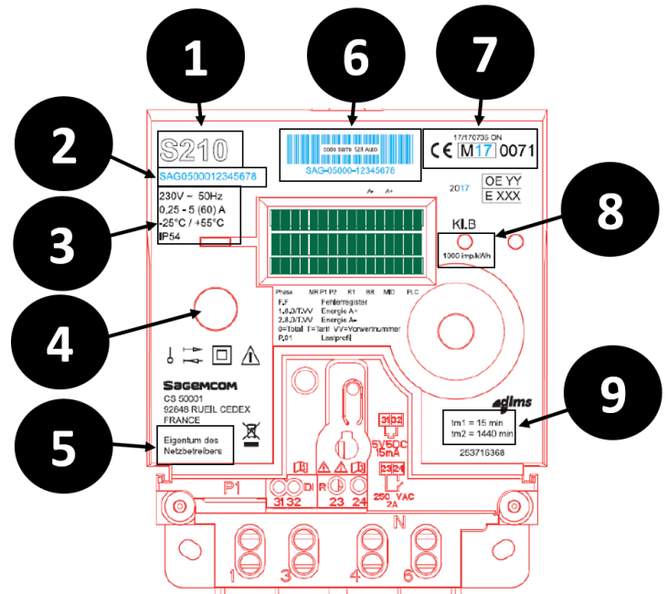
Einphasenstromzähler
