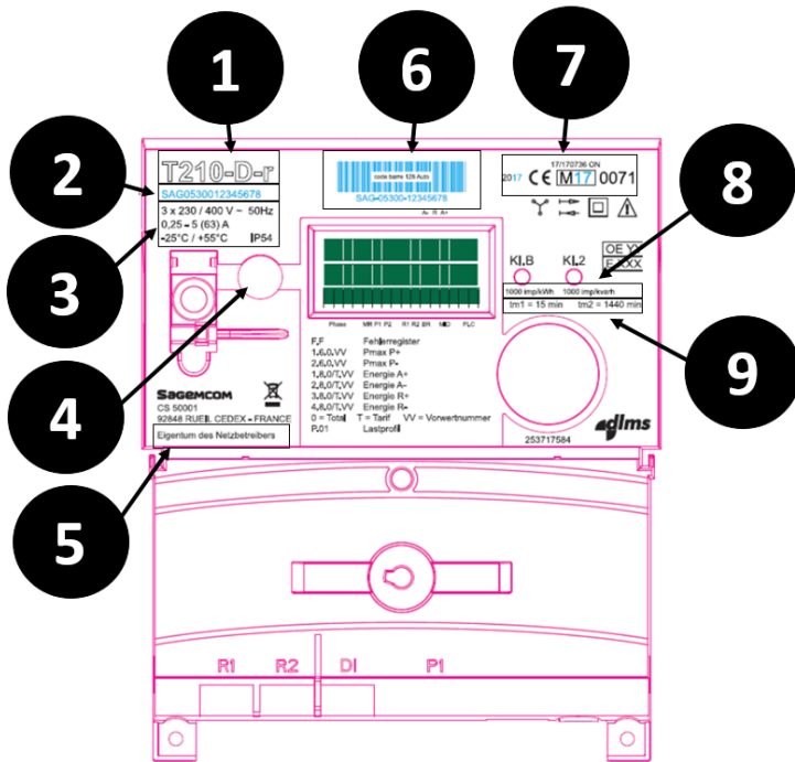
Dreiphasenstromzähler
